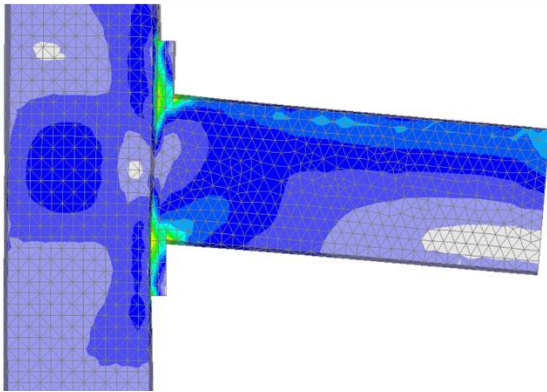
Figura 4 – Incollaggio vs. Contatto. E' evidente come nel caso di esempio l'incollaggio porti a sottostimare sia lo stato di deformazione che lo stress massimo nella flangia.
