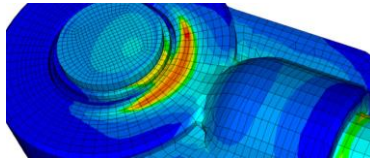
Il comportamento non lineare del materiale nelle analisi FEM
